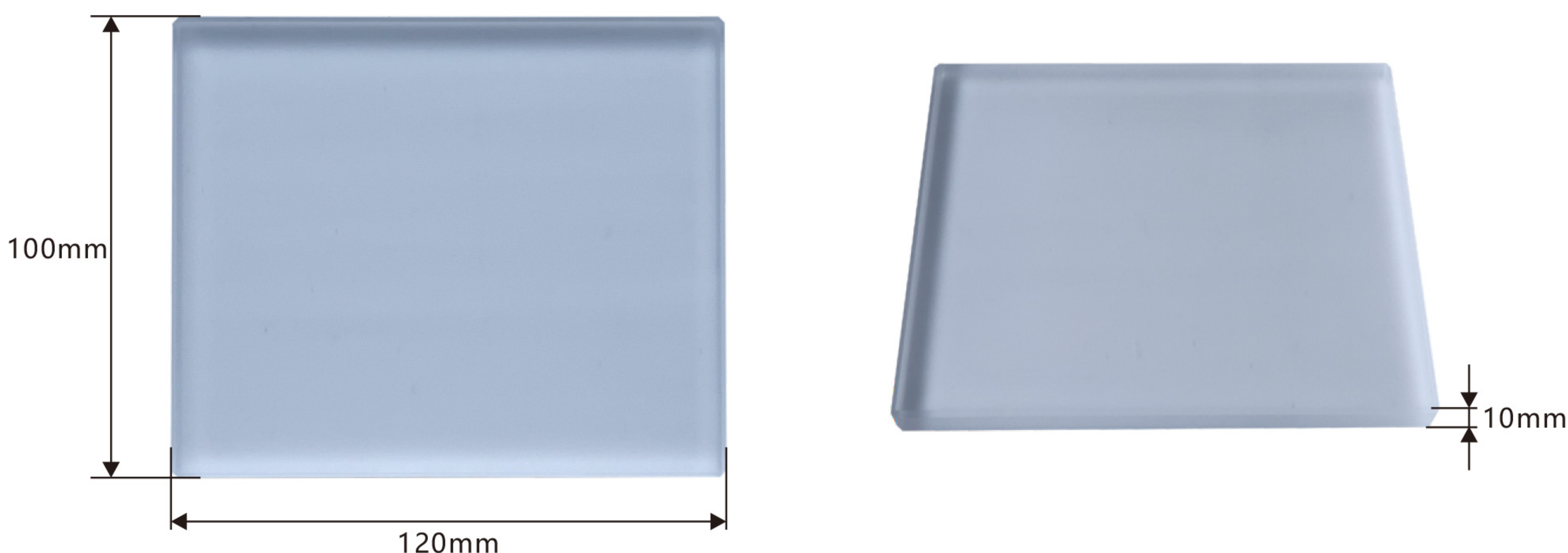
图A.1. 乳腺摄影PMMA模体示意图
