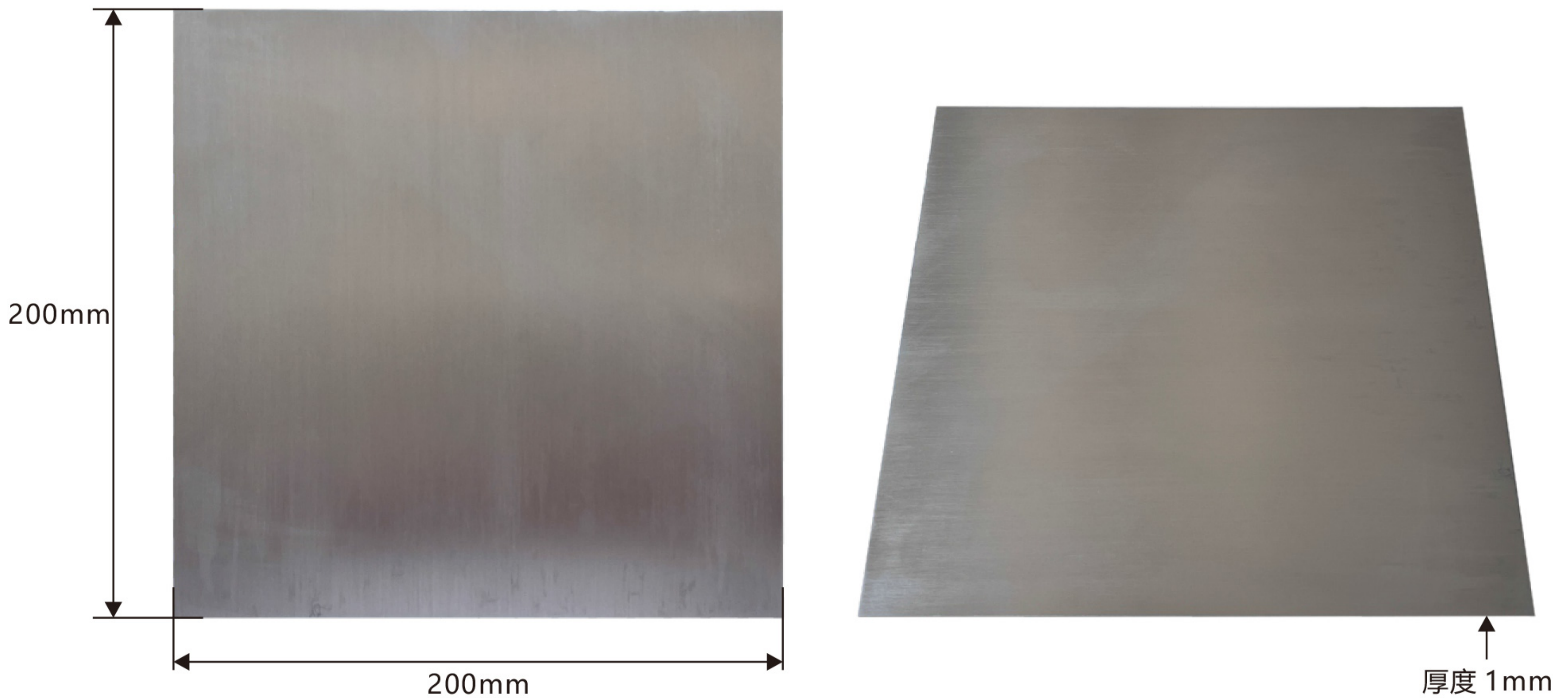
图A.3. 铝板1示意图
